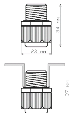
Вариант исполнения с сальниковым вводом
