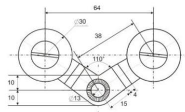
V-образный рычаг
