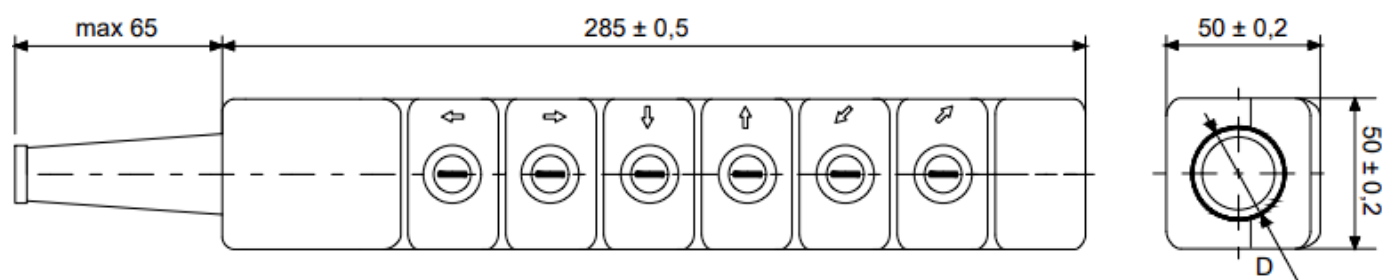
ПКТ-60 У2
