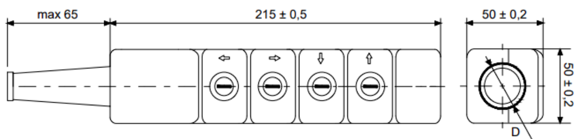
ПКТ-40 У2
