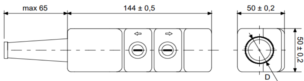
ПКТ-20 У2
