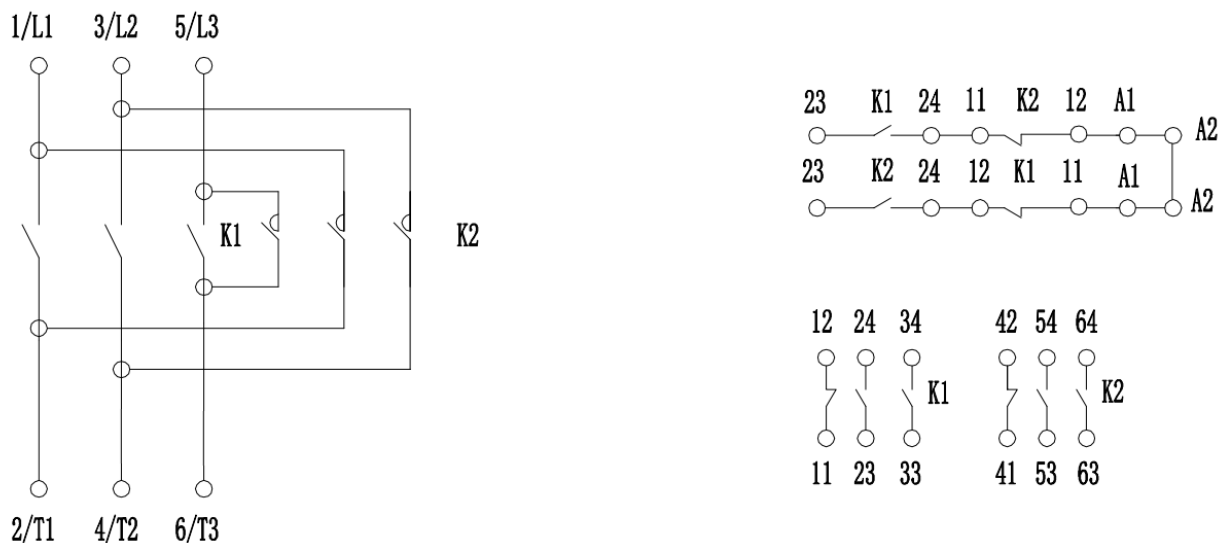
Рисунок 5. Принципиальная электрическая схема реверсивного пускателя ПМ12 100-250А
