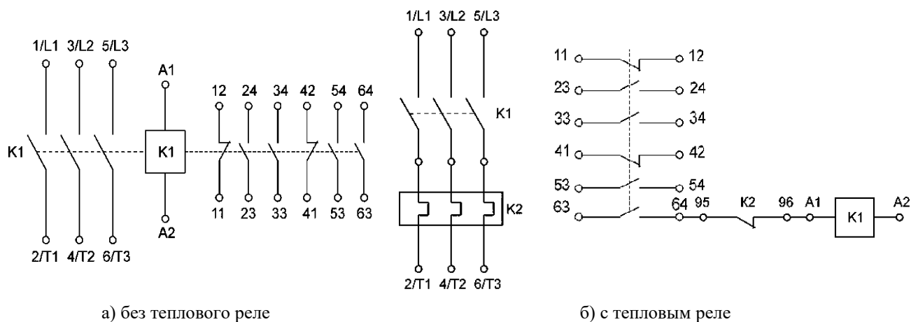
Рисунок 4. Принципиальная электрическая схема пускателя ПМ12 100-250А
