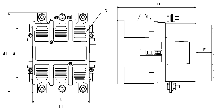
Рисунок 1. Пускатель нереверсивный типа ПМ12-ЭК 100-250А. Степень защиты - IP00
